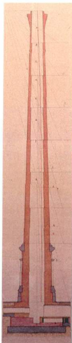
1. Cheminée, épure, décembre 1902 (archives de La Documentation française).
