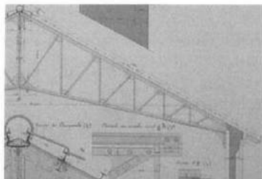
14. Détail du dessin de la charpente métallique de l'atelier C, avril 1903
